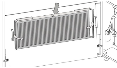
Filter i servicelucka (frånluftsfiler)
