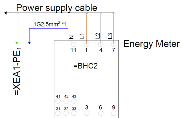
Figur 16: Trefas energimätare
