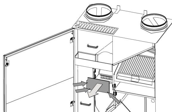
Figur 6: Åtkomst till AQC-L-kontrollboxen i AM 950 F-aggregatet
