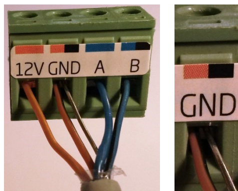
Figur 7: Skärmanslutning
