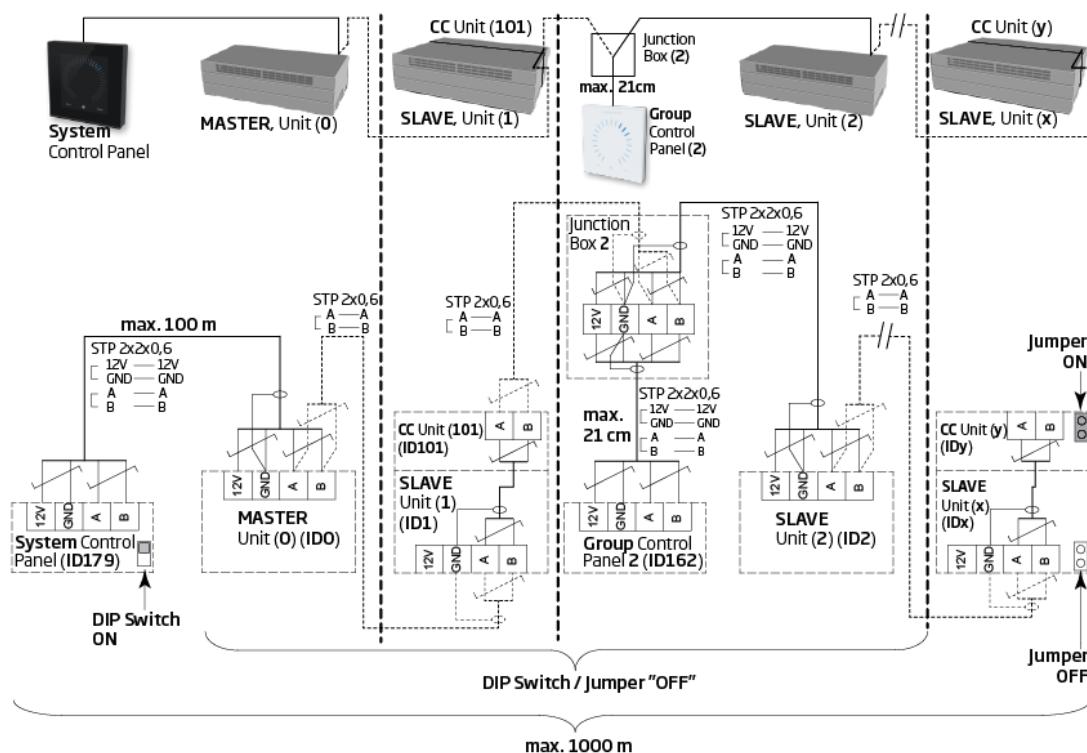
Figur 24: Översikt över installation av Airlinq BMS
