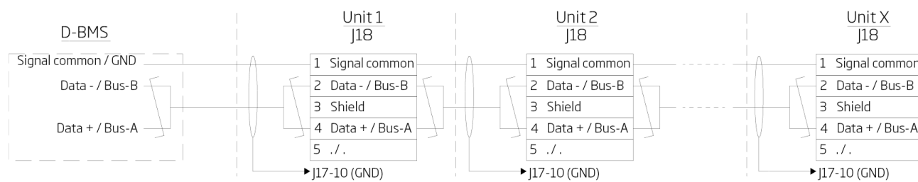
Figur 37: BACnet™ MS/TP, enhetsanslutningar
