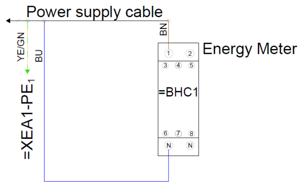
Figur 15: Enfas energimätare
