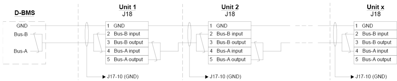
Figur 32: MODBUS®, enhetsanslutningar
