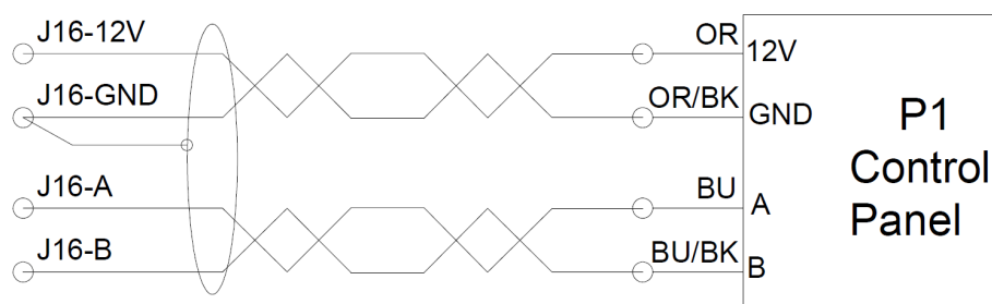
Figur 22: Installation av kontrollpanel, kontrollenhet och panel
