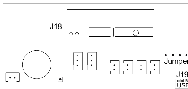
Figur 10: BMS/Ethernet (J18), PC-kommunikation (J19), bygelinställning
